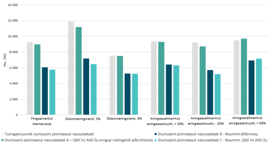
Ilusiliaq 4.7: Malussarissutsimut misissuineq, kingumut nalilernissaanut erniat aningaasaliinermilu aningaasartuutit
