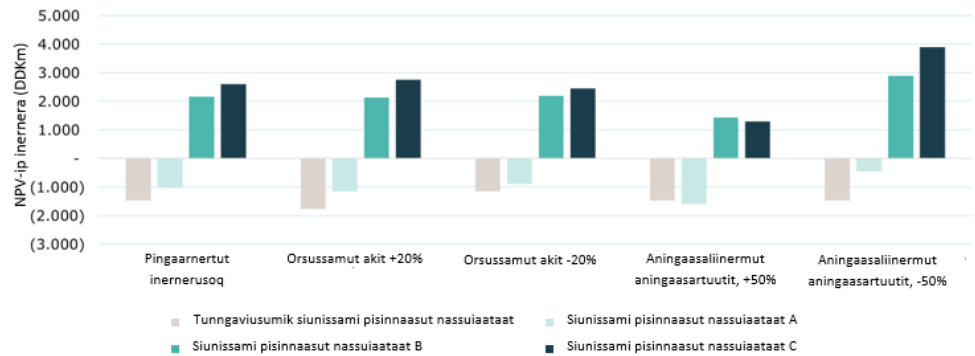
Ilusiliaq 5.3: Malussarissutsimik misissuineq, orussat akii aningaasaliinermullu aningaasartuutit
